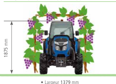
REX3 F - GE CABINE SURBAISSÉE
